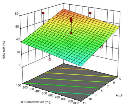
Hình 6 Hiệu quả xử lý độ bằng màu vật liệu PAC
