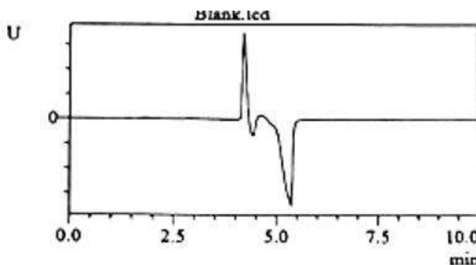
Hình 7 Sắc kí đồ mẫu dung môi
