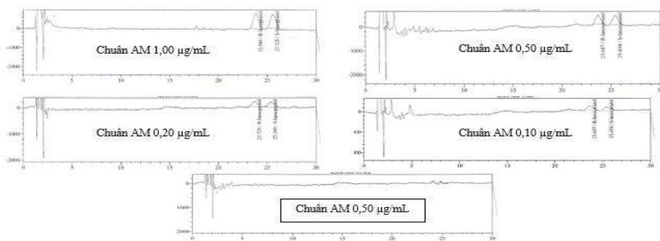
Hình 12 Sắc kí đồ các mẫu chuẩn AM theo nồng độ
