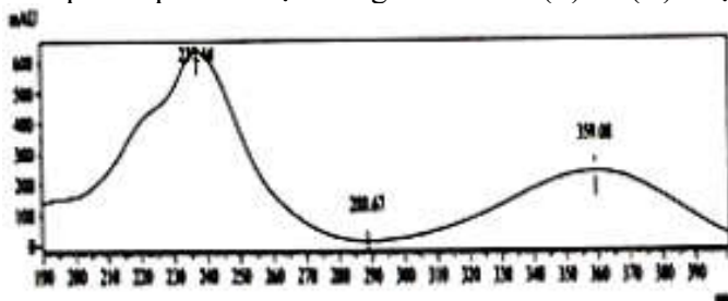
Hình 8 Phổ UV tại thời gian lưu của peak (S)-AM trong mẫu chuẩn
