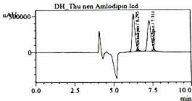
Hình 5 Sắc kí đồ mẫu chuẩn AM
