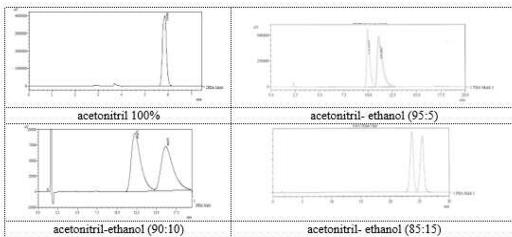
Hình 3 Sắc kí đồ khảo sát khi thay đổi các tỉ lệ pha động khác nhau
